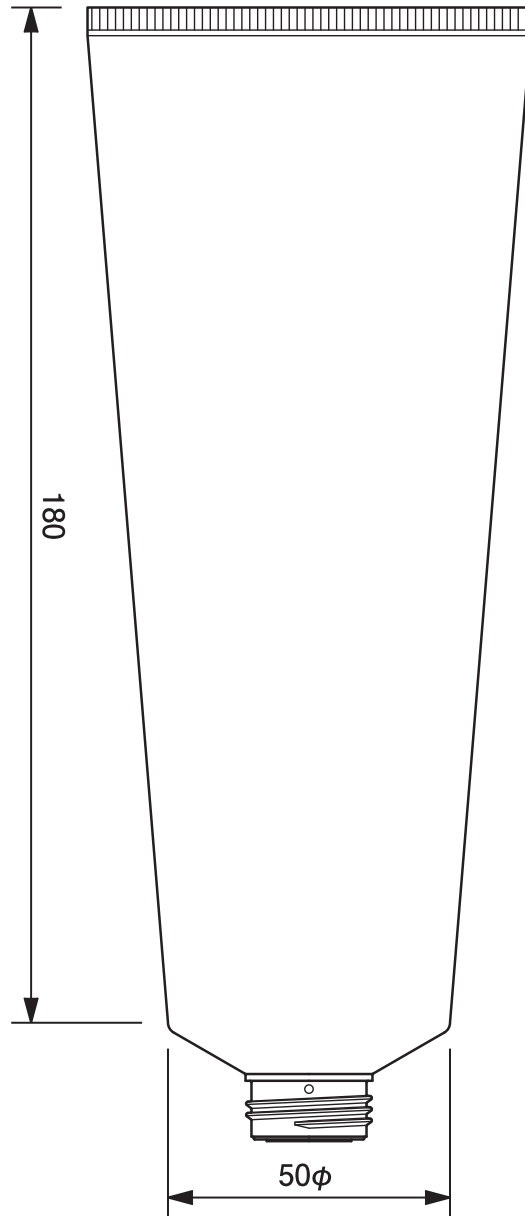
50φチューブ平ネジ用 -277 50mm dia. Tube-277
