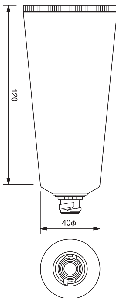
40φII ワンタッチチューブ -114 40mm dia. Flip-top Cap Tube-114
