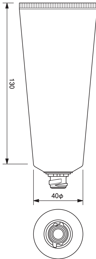
40φII ワンタッチチューブ -124.6 40mm dia. Flip-top Cap Tube-124.6
