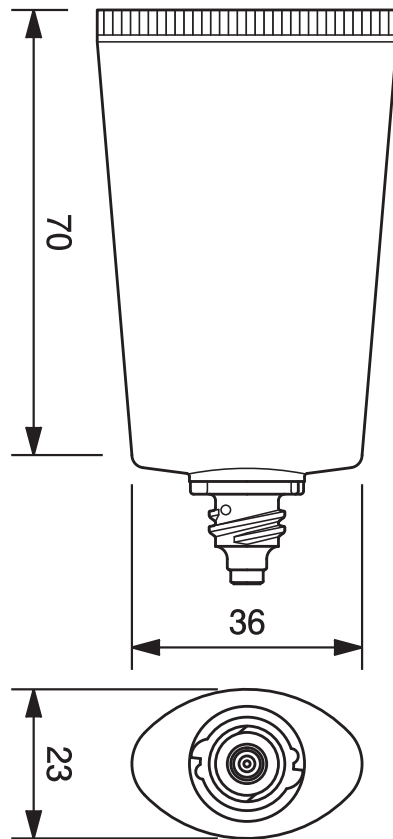
30φオーバルチューブ -30.7 30mm dia. Oval Tube-30.7
