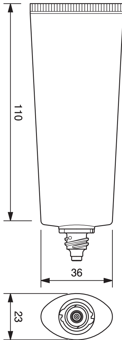
30φオーバルチューブ -57.3 30mm dia. Oval Tube-57.3
