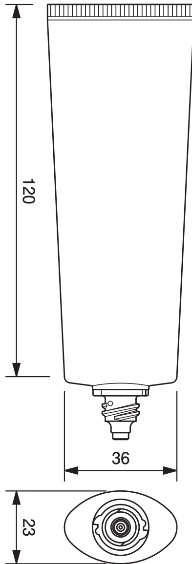
30φオーバルチューブ -63 30mm dia. Oval Tube-63
